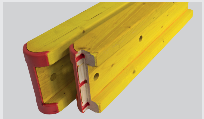
Gesamte Stirnseite geschützt durch schlagfeste Schutzkappe für hohe Einsatzzahlen und lange Lebensdauer.
