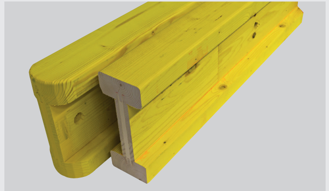
Steg aus 3-Schichtplatten mit keilverzinkten Gurtanschlüssen für hohe Stabilität und Langlebigkeit bei Holzträger PF20 und H20 top.
